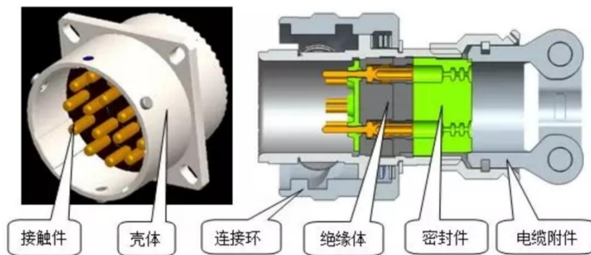
图13：连接器基本构成
