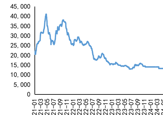
图15：环氧树脂价格走势（元/吨）
