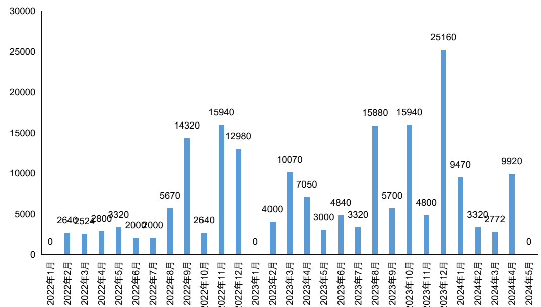
图27：煤电月度开工容量（MW）
