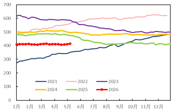
图 15：美国原油钻机数（台）
