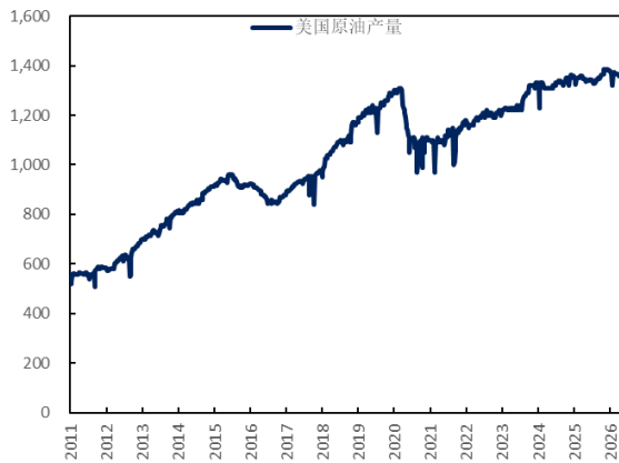
图 12：美国原油产量（万桶/天）
