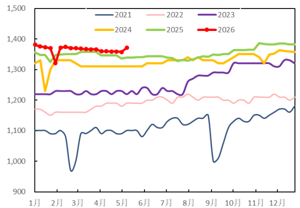
图 13：美国原油产量（万桶/天）
