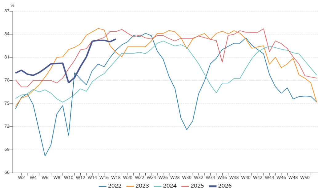
图12、高炉开工率
