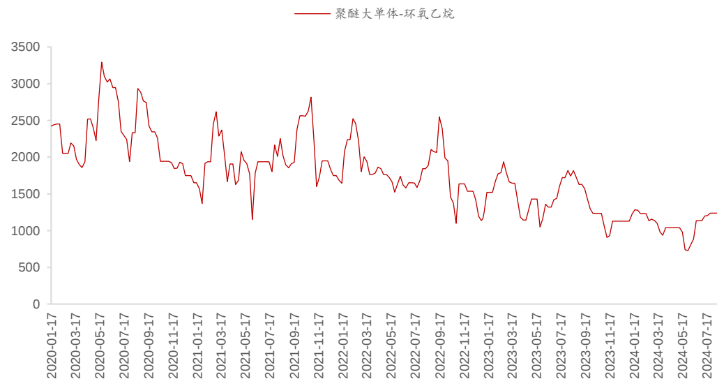
图表 25 聚醚大单体-环氧乙烷价差走势图（元/吨）
