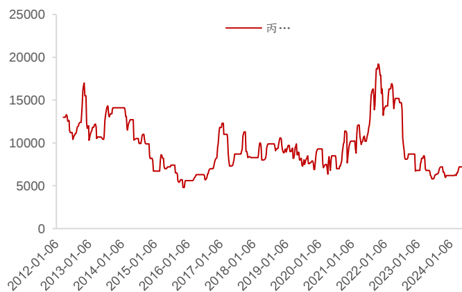
图表 10 丙烯酸价格走势图（元/吨）
