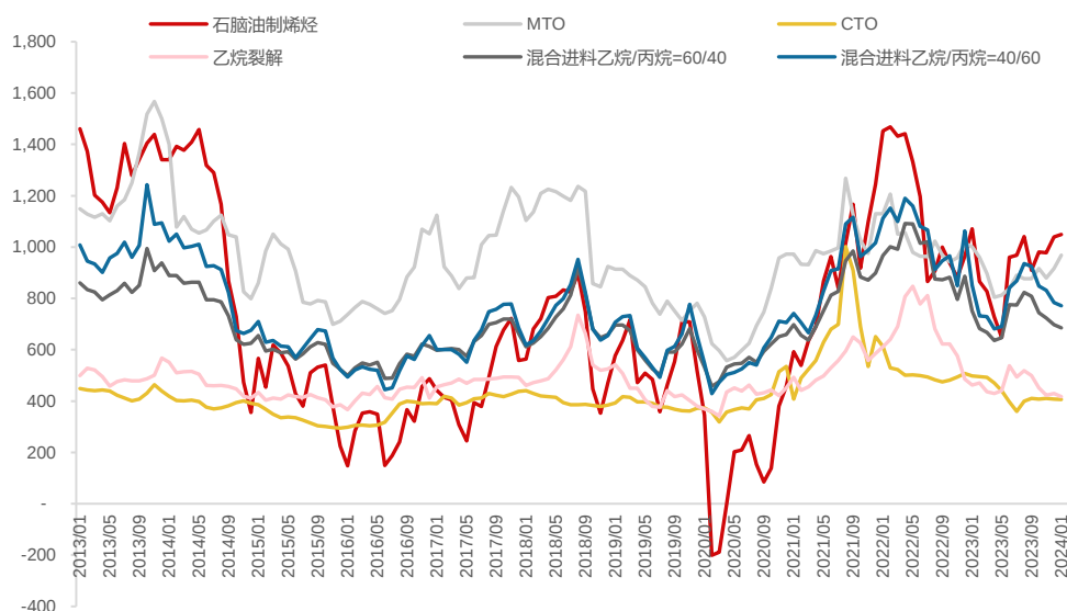
图表 35 现金成本（美元/吨）
