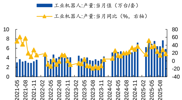
图 11：我国工业机器人产量及同比变化情况
