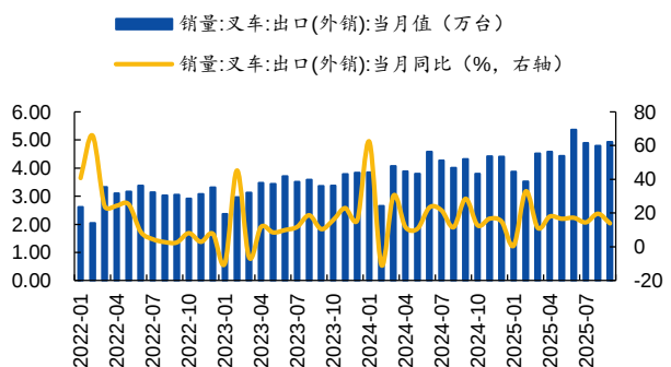
图 13：我国叉车出口数量及同比变化情况
