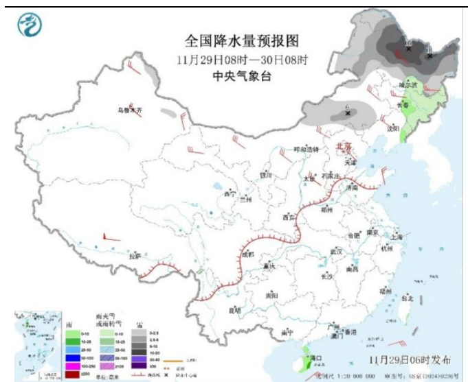
图5：11月末我国北方地区持续降雪降温
