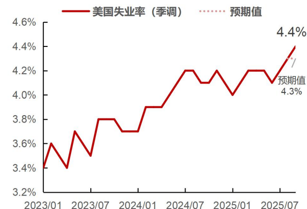
图表 9：美国失业率情况
