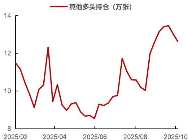
图表 19: COMEX 其他多头持仓情况
