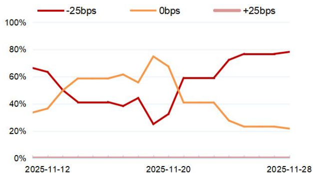
图表 14：2025 年 12 月 FOMC 单月利率变动概率
