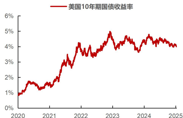
图表 17: 美国 10 年期国债收益率情况
