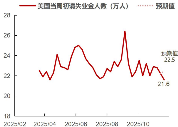
图表 11：美国当周初请失业金人数情况
