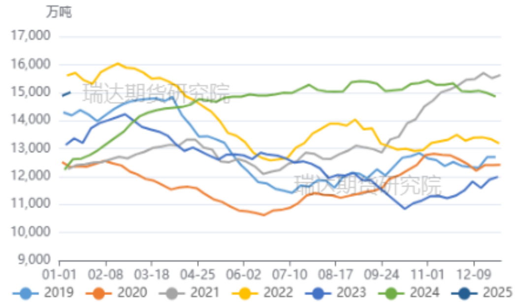
图23、库存：铁矿石
