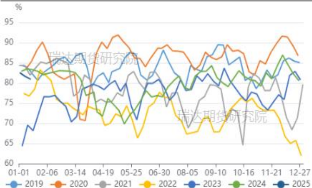
图18、PTA开工率
