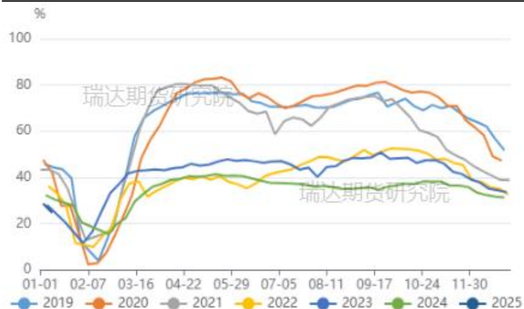
图14、水泥发运率
