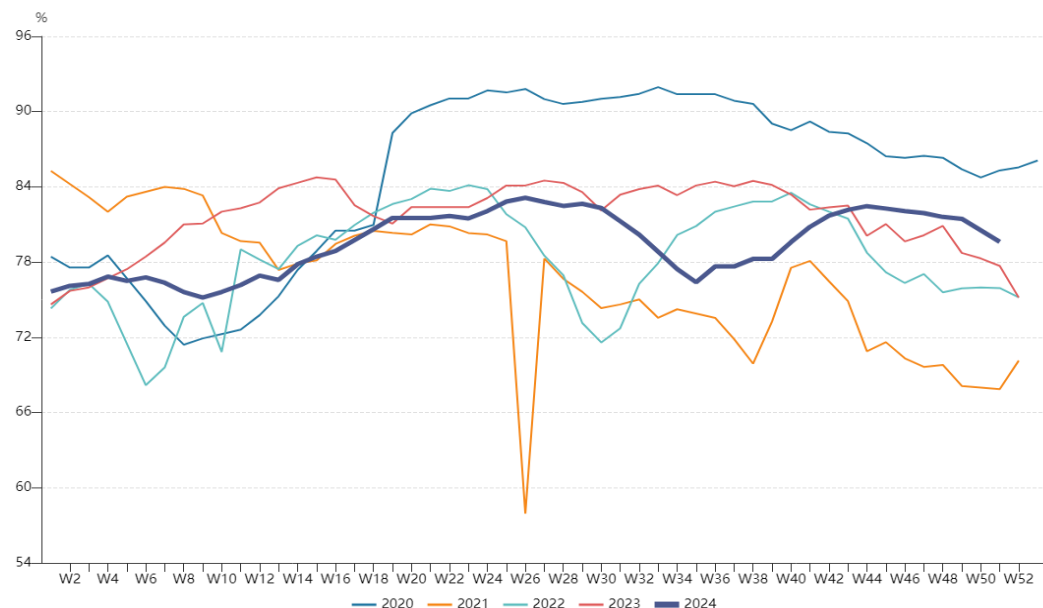
图12、高炉开工率
