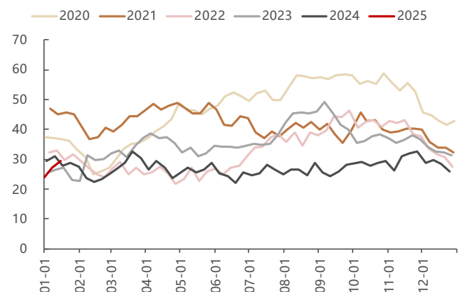
图8：石油沥青装置开工率上升 (%)
