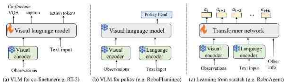
图 13 (网络版彩图) LLM/VLM 驱动的基础策略基本结构
