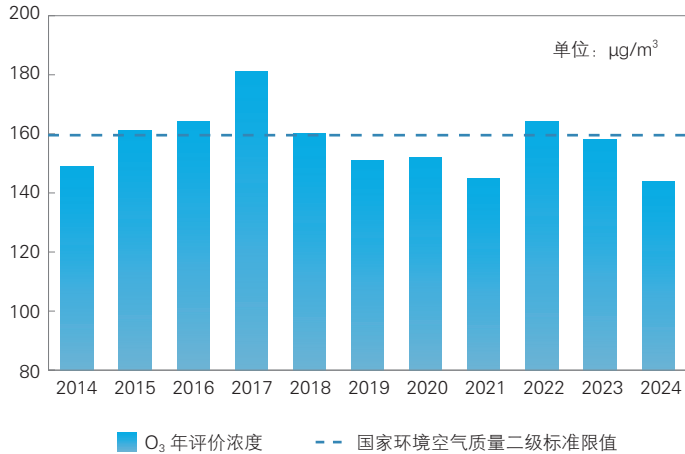
图 3-3 2014-2024 年上海市 O 3 年评价浓度变化趋势
