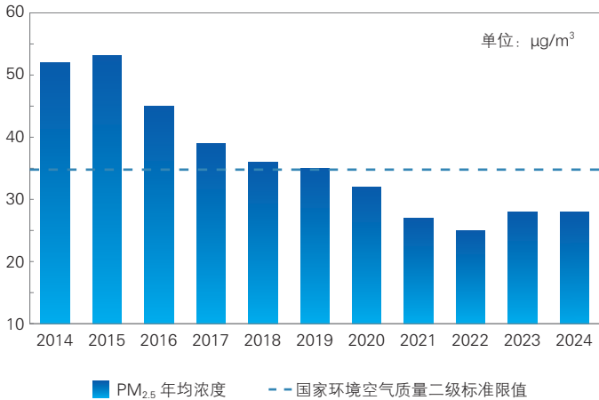
图 3-2 2014-2024 年上海市 PM 2.5 年均浓度变化趋势
