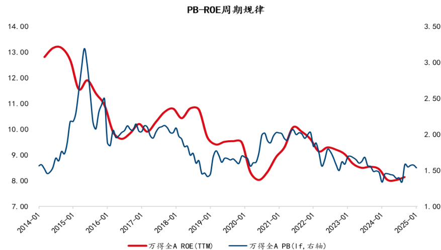
图：全A、沪深300近10年PB-ROE轨迹
