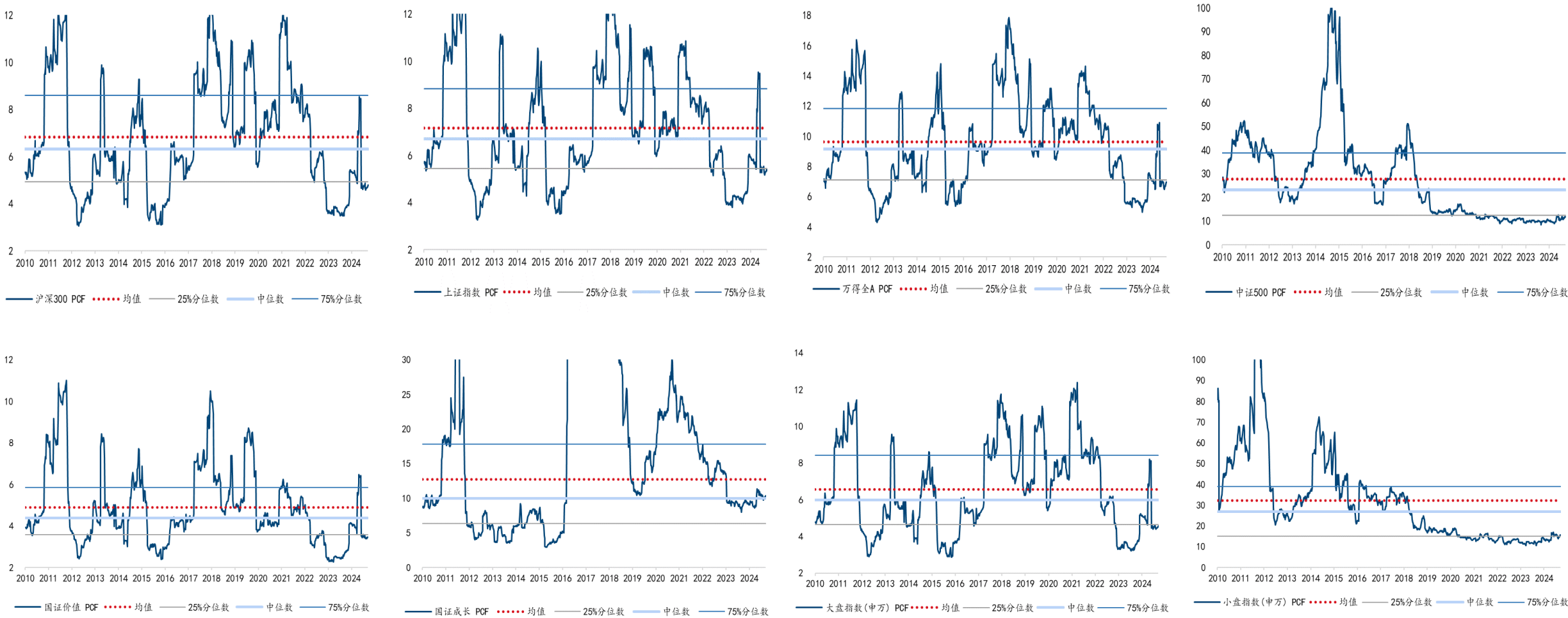
图：A股宽基指数PCF长序列对比
