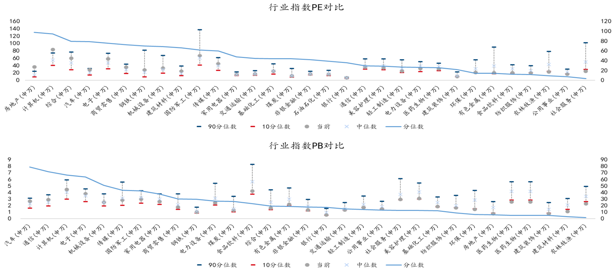
图: 行业指数长期估值对比 (PE、PB)
