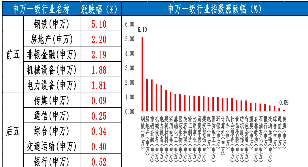
图表 3 申万 I 级行业日涨跌幅情况 (%) (2025. 02. 26)
