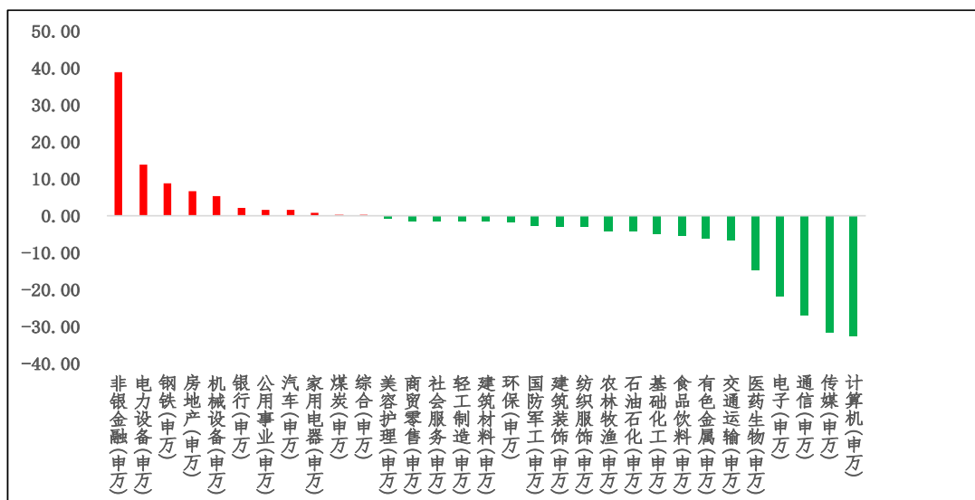
图表 4 申万 I 级行业日主力资金净流入 (亿元) (2025. 02. 26)
