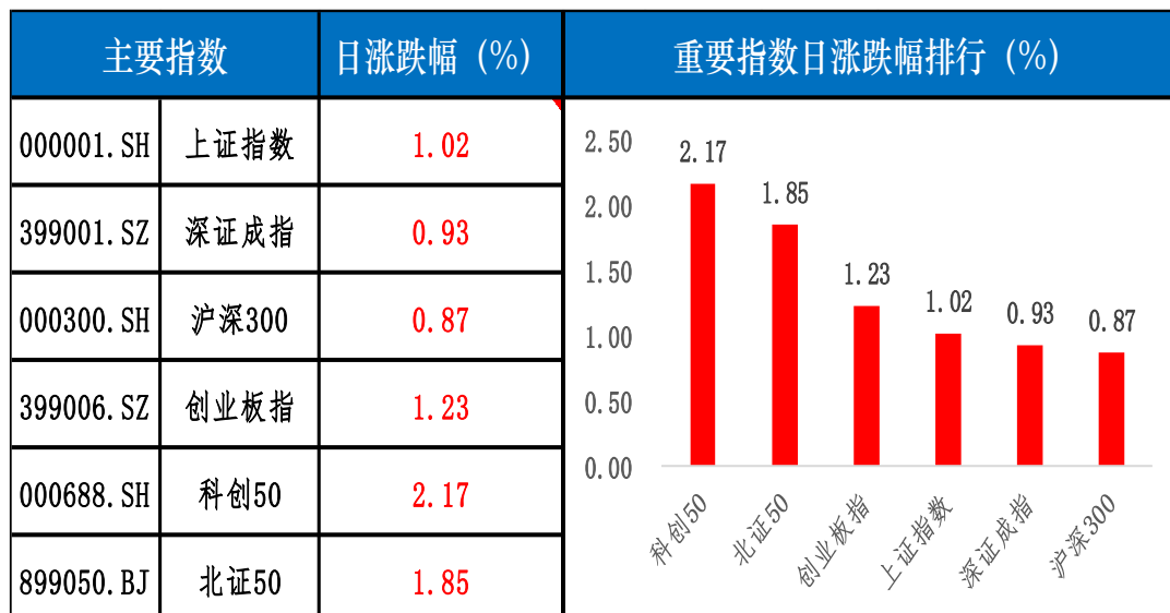
图表 1 重要指数日涨跌幅 (%) (2025.02.26)
