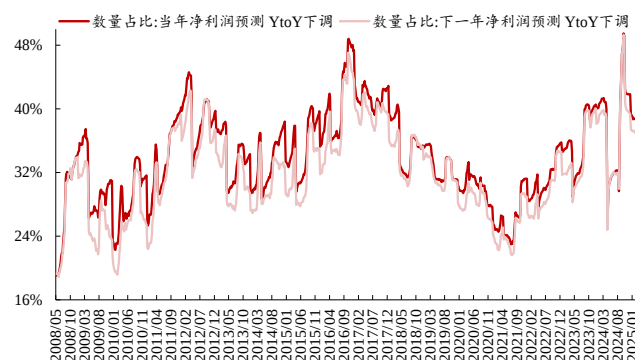
图18: 上周 (20250224-20250228) 全 A 中 2025/2026 年净利润预测下调(相较于最近一期财报前的预测)的个股比例相较于上一期均上升
