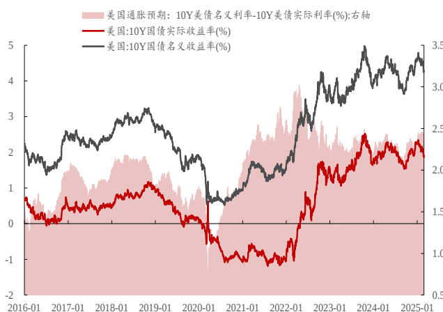
图4：上周(20250224-20250228)10Y 美债名义/实际利率均下降，其背后隐含的是通胀预期回落
