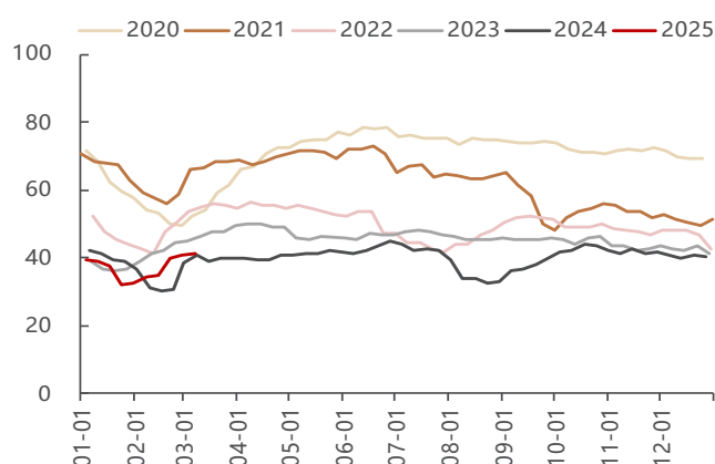
图1：螺纹钢主要钢厂开工率较上周上升（%）
