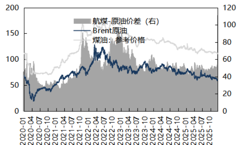
原油、国内航煤价格及价差（美元/桶，美元/桶）
