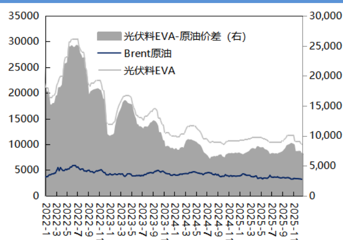
原油、EVA光伏料价格及价差（元/吨，元/吨）
