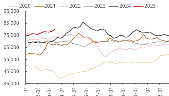
图24：无氧铜杆价格上升（元/吨）
