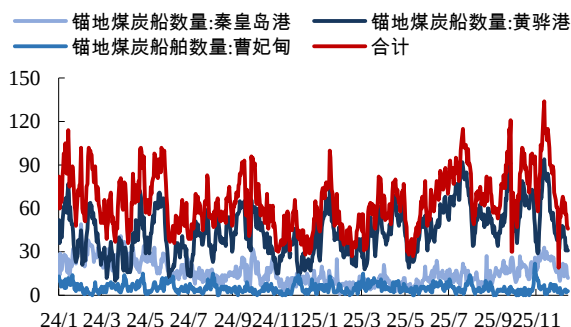
图12：12月三港合计锚地船舶数量月环比下降59.29%（艘）
