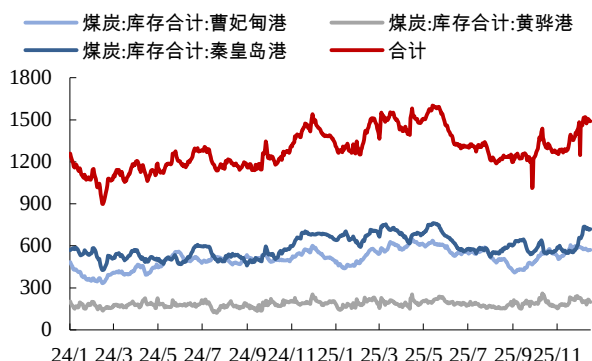
图11：12月三港合计煤炭库存量月环比上升15.58%（万吨）
