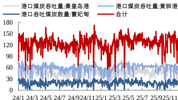
图10：12月三港合计吞吐量月环比下降20.29%（万吨）
