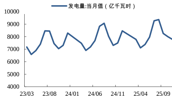
图16：11月发电 7792.02 亿千瓦时，同比增长 3.96%
