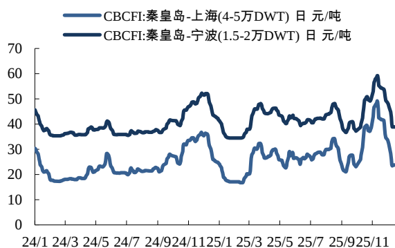
图19：12月国内航线 CBCFI 月环比下跌
