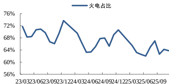
图18：11月火电占发电的比重达 63.78%，同比下降 5.26%
