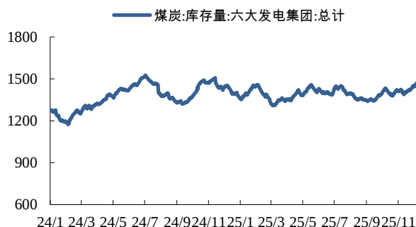
图14：12月六大发电集团库存量月环比上升0.40%
