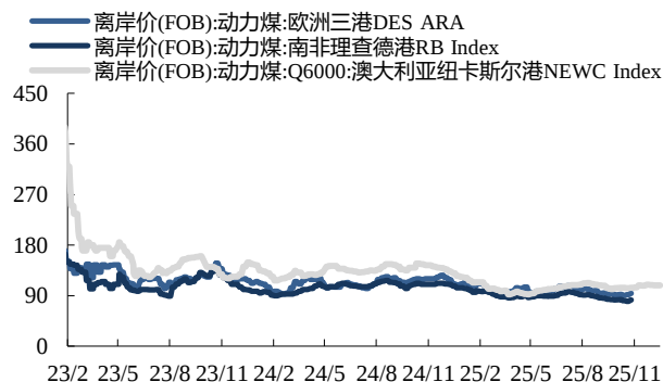
图4：国际动力煤离岸价情况（美元/吨）
