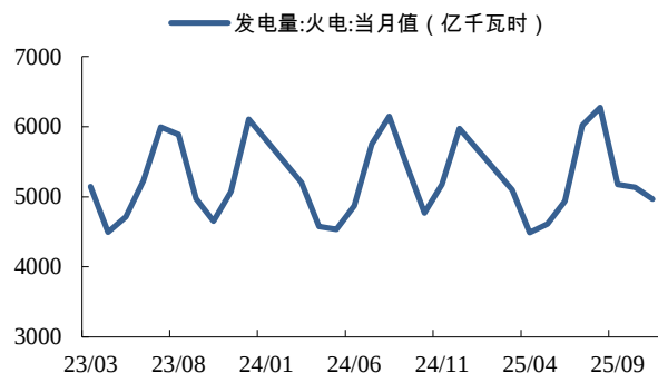
图17：11月火电发电 4969.52 亿千瓦时，同比下降 3.97%
