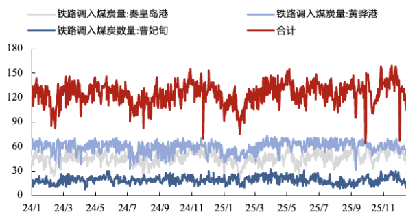
图9：12月三港合计铁路调入量月环比下降32.80%（万吨）
