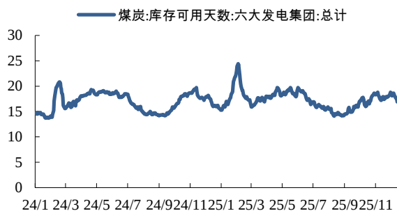
图13：12月六大发电集团库存可用天数月环比下降3.43%
