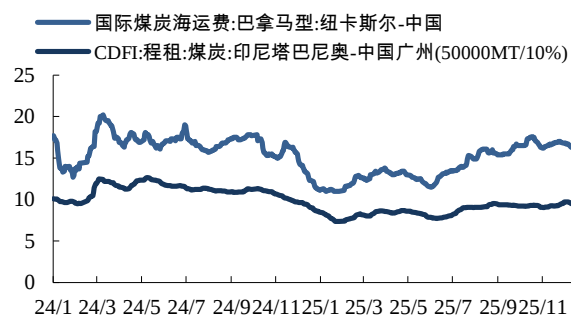
图20：12月国际海运费涨跌不一（单位：美元/吨）
