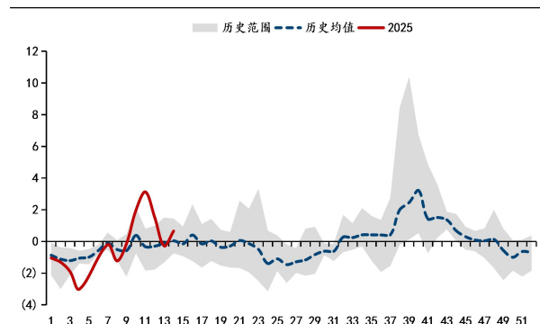
图25: 水泥价格指数: 全国 (环比增速)
