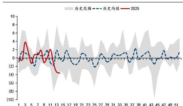
图23: 现货结算价:LME 铝 (环比增速)
