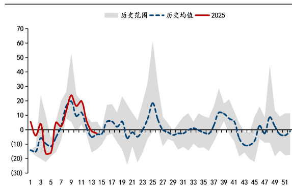
图32: 波罗的海干散货指数(BDI)(环比增速)
