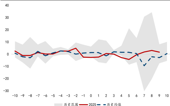
图35: 期货结算价(连续):布伦特原油（环比增速）
