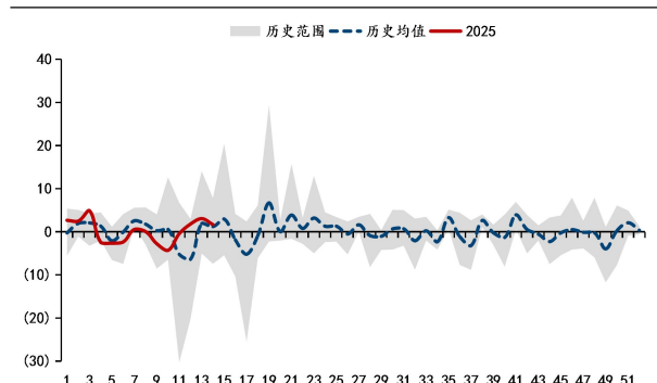
图21: 期货结算价(连续):布伦特原油（环比增速）
