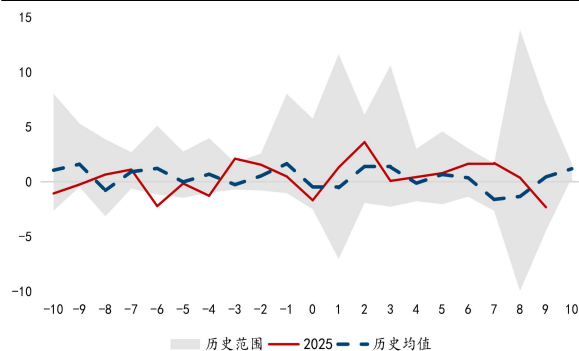
图34: 现货结算价:LME 铜（环比增速）
