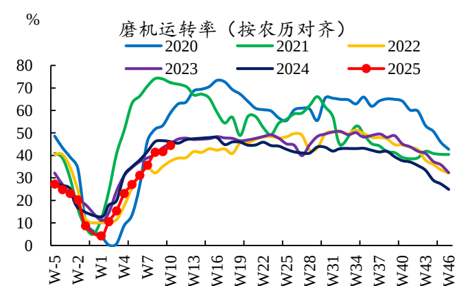
图2：磨机运转率季节性位置有所回升
