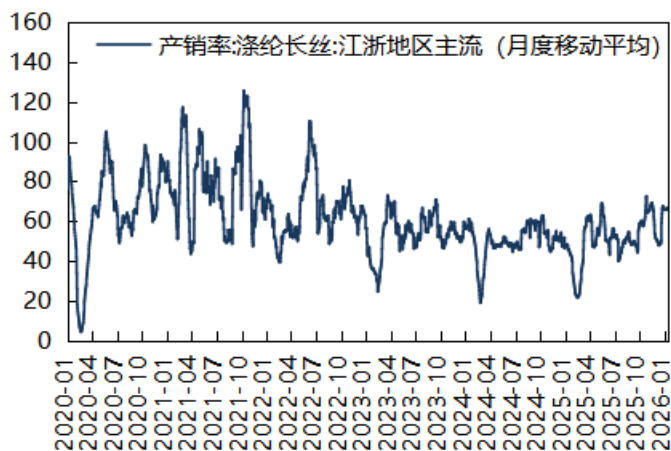
江浙地区涤纶长丝产销率 (%)
