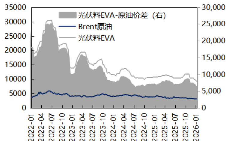
原油、EVA光伏料价格及价差（元/吨，元/吨）
