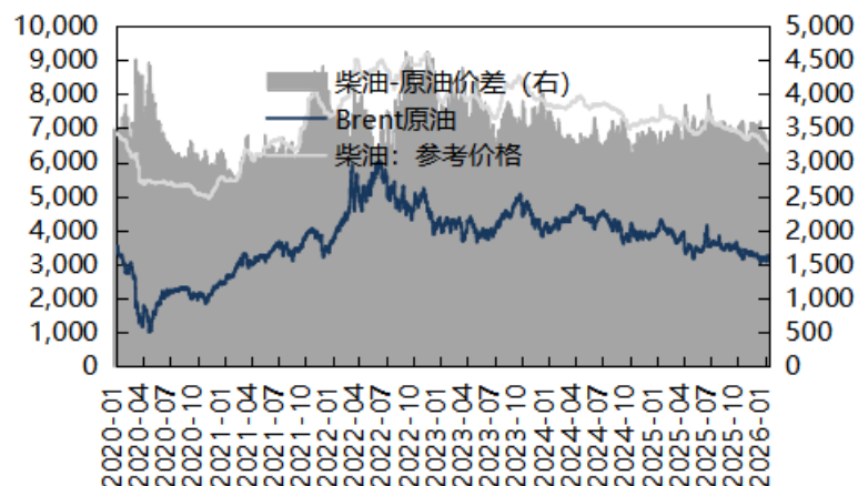
原油、国内柴油价格及价差（元/吨，元/吨）
