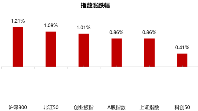
图2：指数涨跌幅
