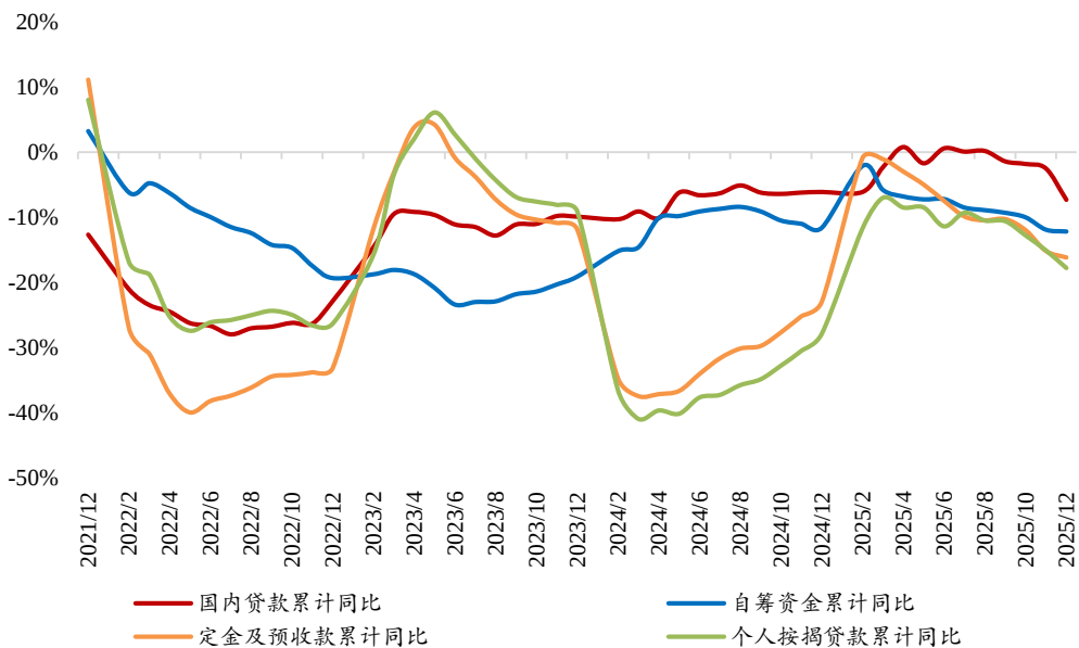
图8：2025 年 1-12 月国内贷款、自筹资金、定金及预收款、个人按揭贷款累计同比分别-7.3%、-12.2%、-16.2%、-17.8%
