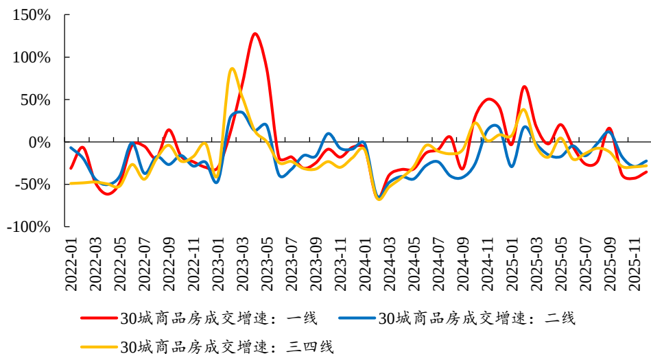
图4：2025 年 12 月 30 大中城市中一、二、三四线城市商品房成交面积增速分别同比-35.3%、-22.4%、-28.0%
