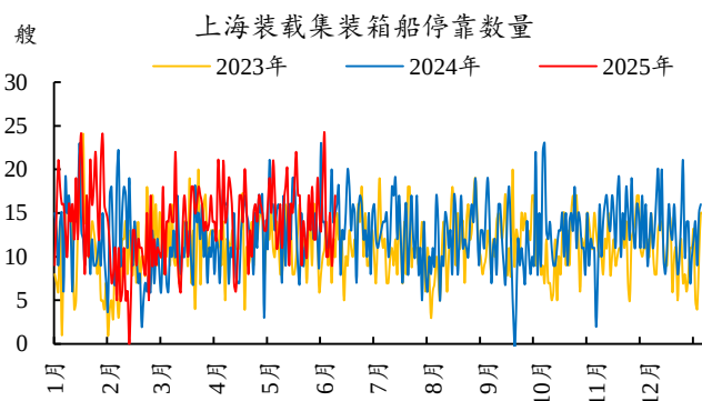
图37：上海装载集装箱船停靠数量近期明显回落
