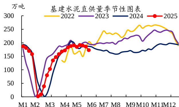
图4：基建水泥直供量显著回落
