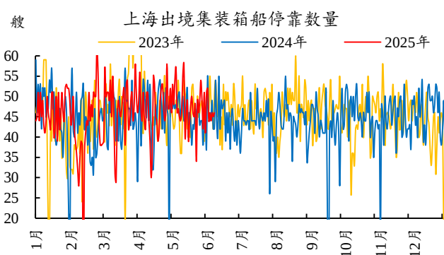
图38：上海出境集装箱船停靠数量近期明显回落
