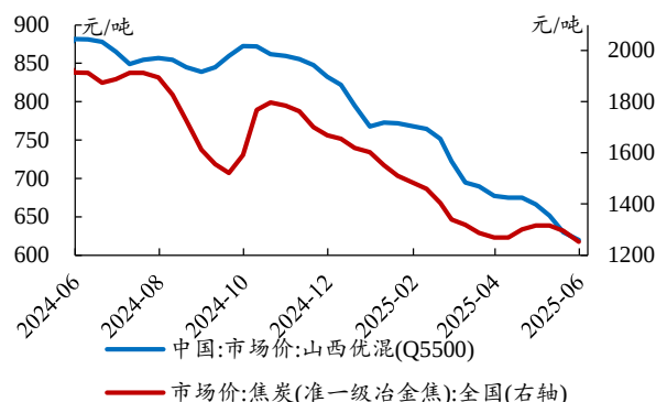
图22：最近两周焦炭价格有所回落
