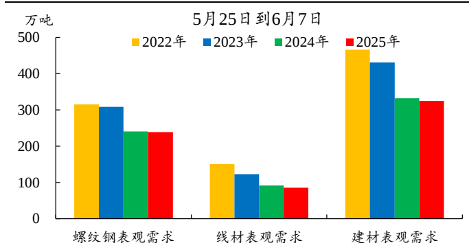
图11：建材需求弱于历史同期
