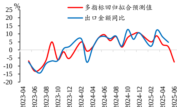
图34：根据截至6月8日数据，预计6月出口同比或将在-8%左右
