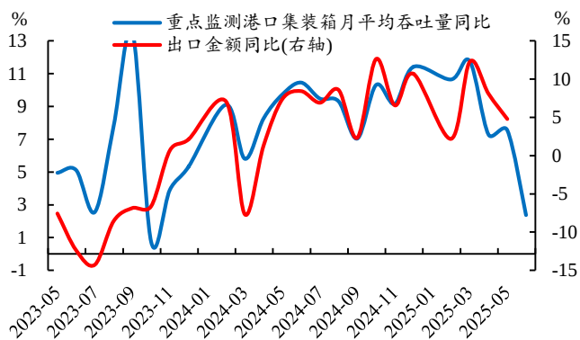
图33：集装箱吞吐量指向6月出口大幅回落
