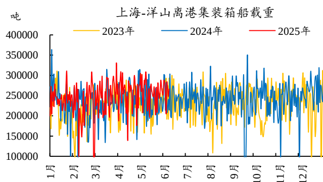
图40：上海-洋山离港集装箱船载重并未大幅回升
