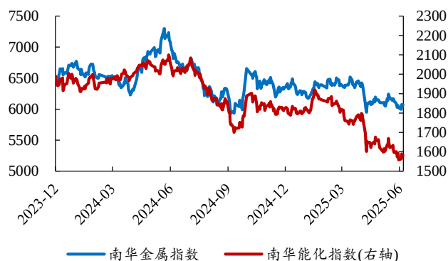
图20：最近两周南华能化指数震荡偏弱运行
