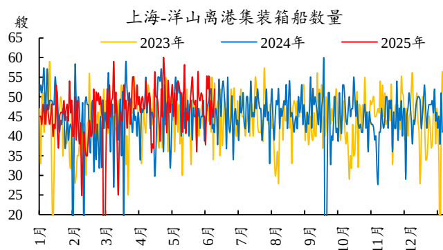
图39：上海-洋山离港集装箱船数量震荡运行
