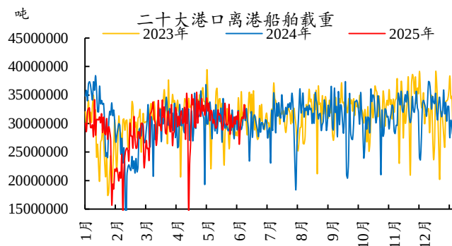
图36：离港船舶载重并未大幅回升
