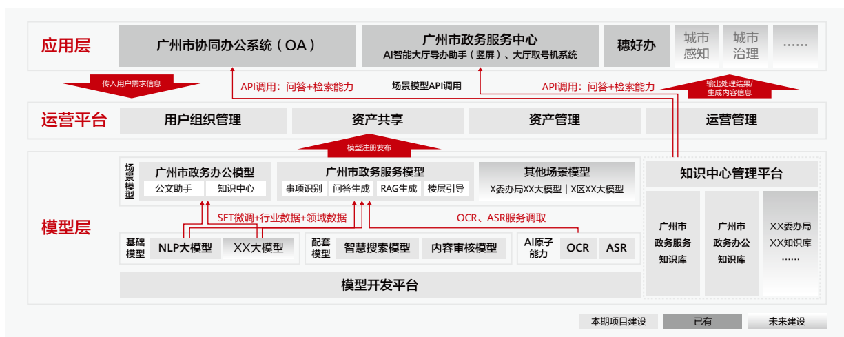
图 25 模型架构图
