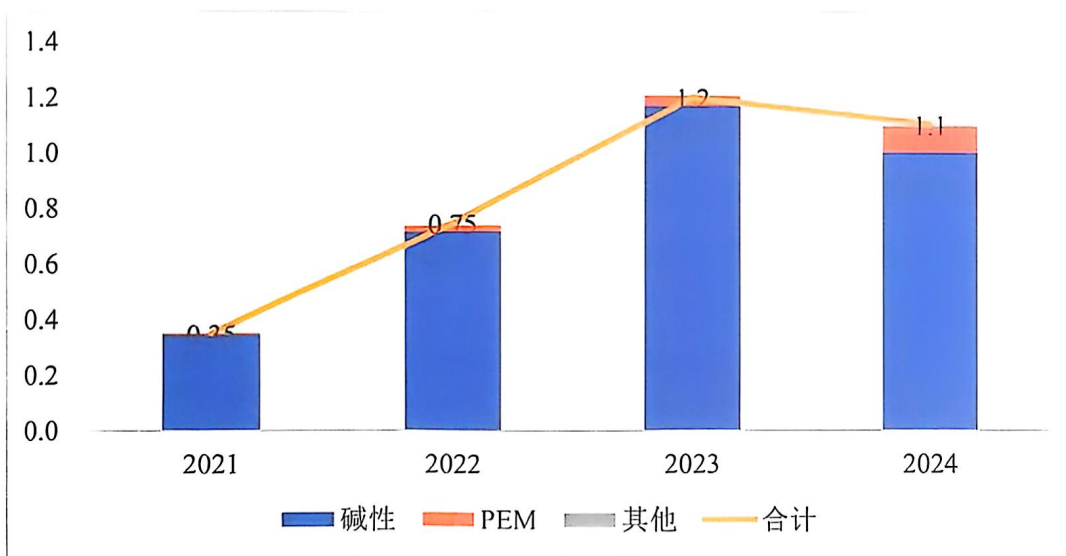
图表 28 2021-2024 年中国电解槽出货量（单位：GW）
