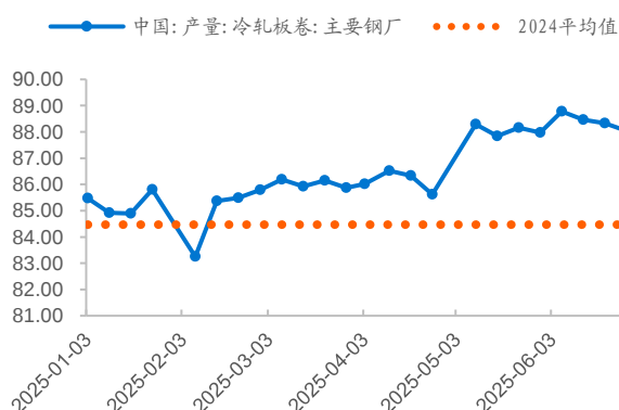
图30 冷轧板卷产量
