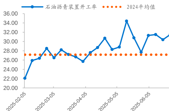
图7 石油沥青装置开工率 (%)
