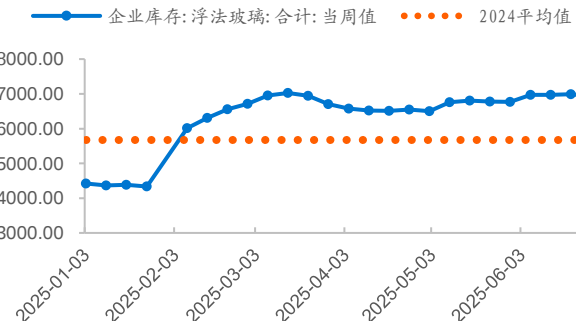
图20 浮法玻璃库存（万重量箱）
