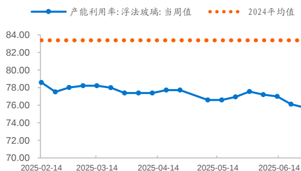
图26 浮法玻璃产能利用率 (%)
