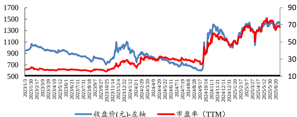
图13：北证 50 指数 PE TTM67.21X
