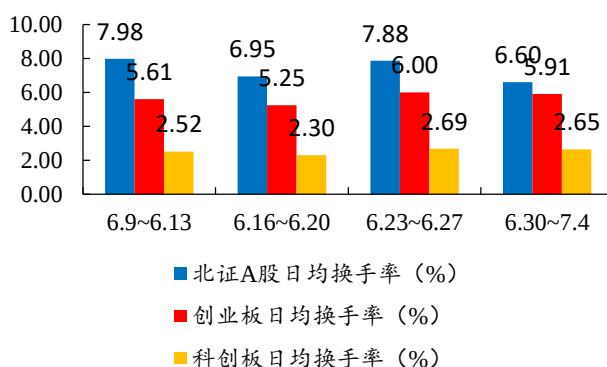
图12：北证 A 股本周日均换手率 6.60% (-1.28pcts)
