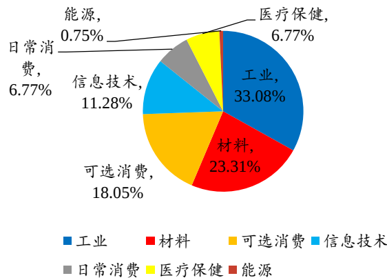
图2：新受理企业中工业企业占比 33.08%
