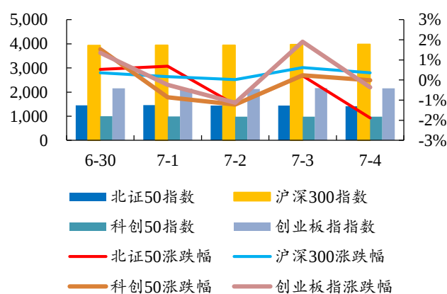
图15：本周创业板、沪深 300 较上周相比出现上涨
