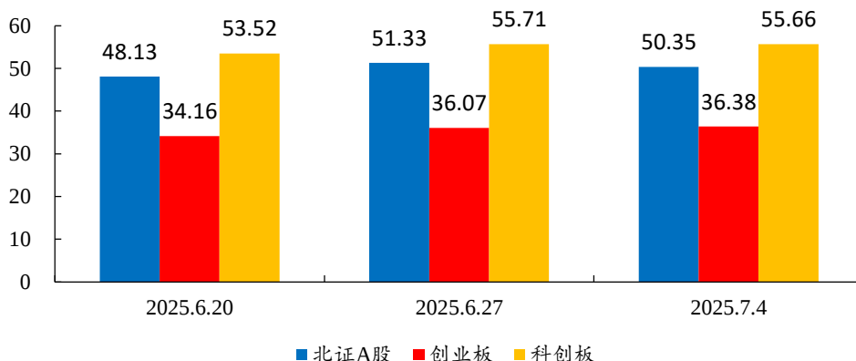
图10：本周北证 A 股整体 PE 估值增长到 50.35X
