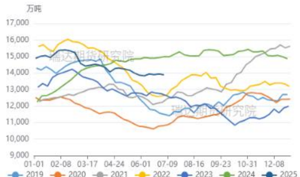
图21、库存：铁矿石
