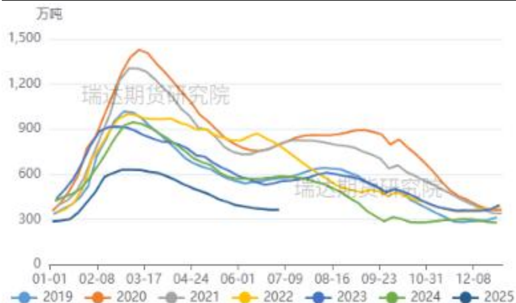
图20、库存：螺纹钢
