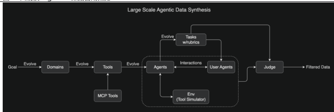
图2: 大规模 Agentic 数据合成概览
