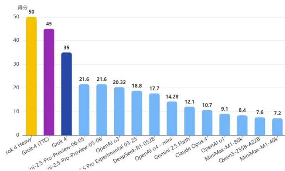
图1：HLE 大模型得分排行榜
