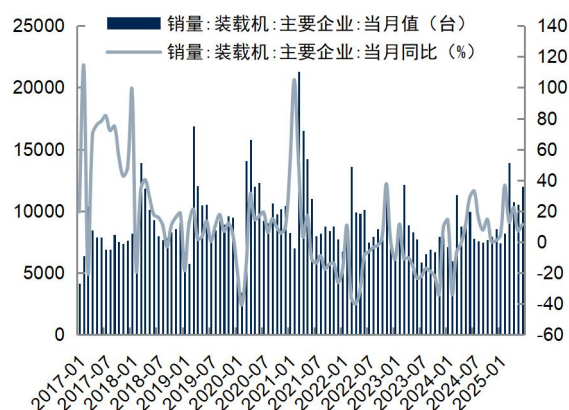
图28: 2025 年 6 月装载机主要企业销量同比增长 11.30%
