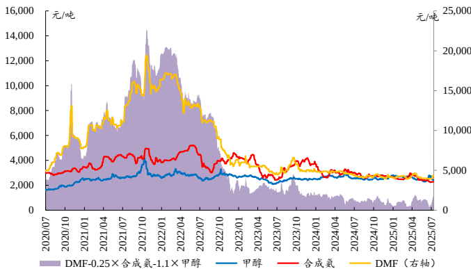
图42：本周 DMF 价差扩大
