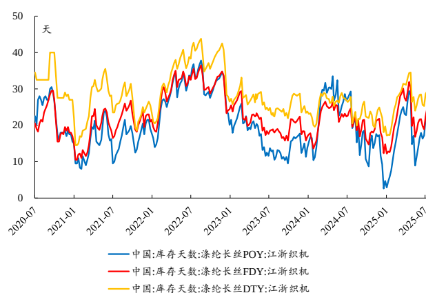
图4：本周涤纶长丝 POY 库存天数增加
