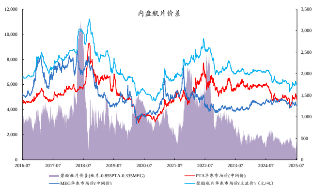
图32：本周瓶片价差扩大
