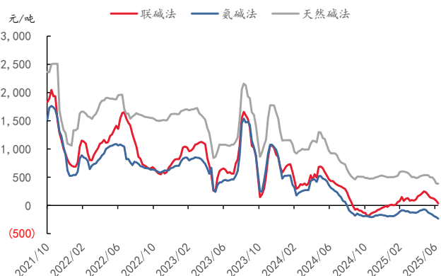
图表42：各工艺路线盈利情况
