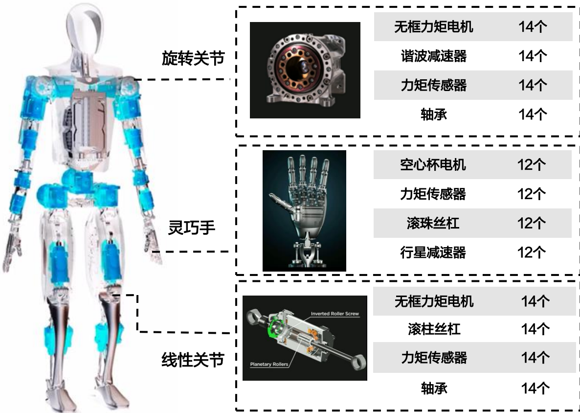
图：特斯拉Optimus机械部件拆解
