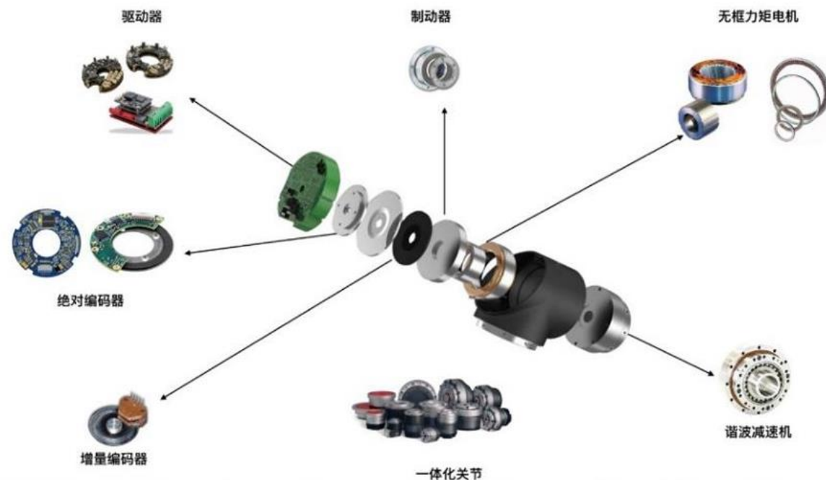
图：一体化关节中使用无框力矩电机
