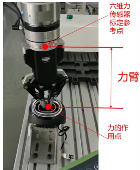
图：六维力传感器在机器人末端使用
