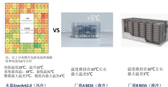
图表 21：液冷比风冷效果更好
