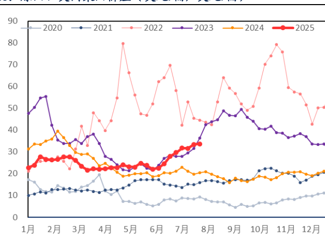
图 20: 原油、美国柴油价差 (美元/桶, 美元/桶)
