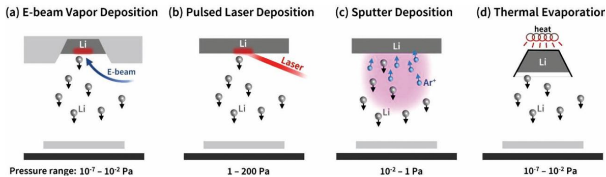
图37：四种常见的气相沉积法制备锂金属负极
