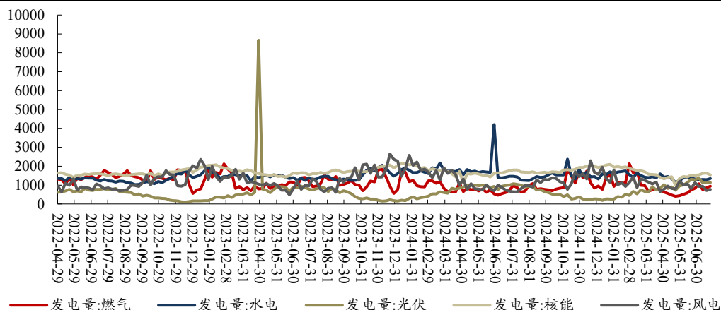
图7: 最近一年欧洲发电结构 (GWh/日, 周度数据, 截至 2025/7/25)
