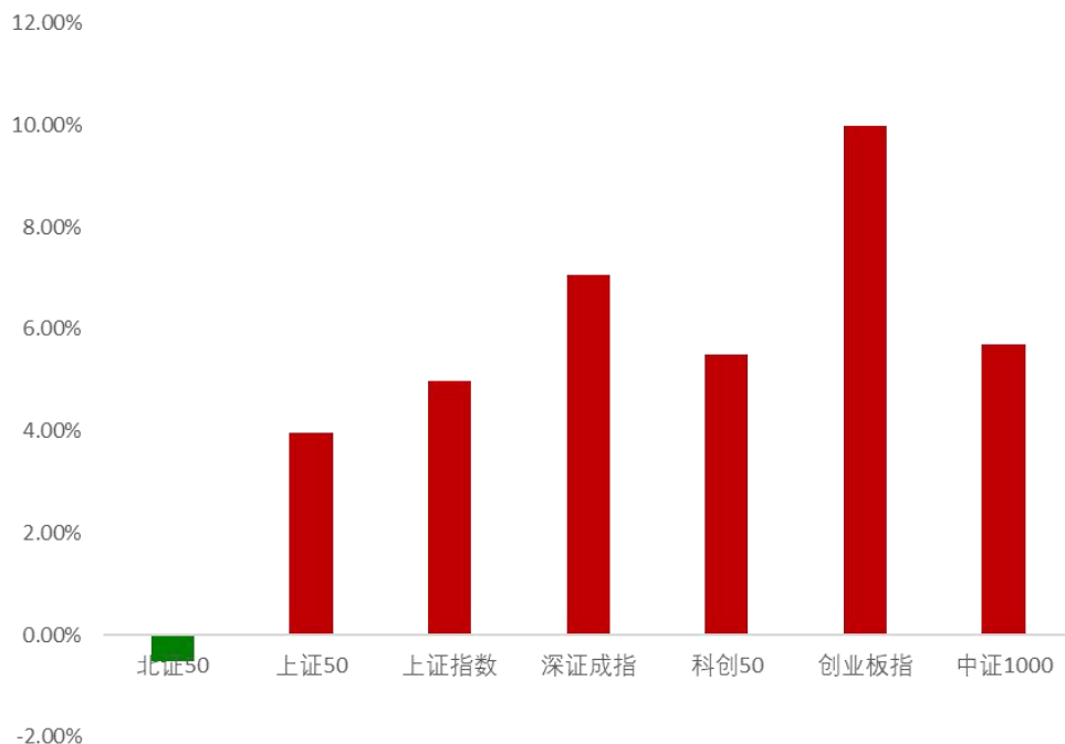
图 1：北证 50 近一月行情走势（截至 2025 年 7 月 30 日）
