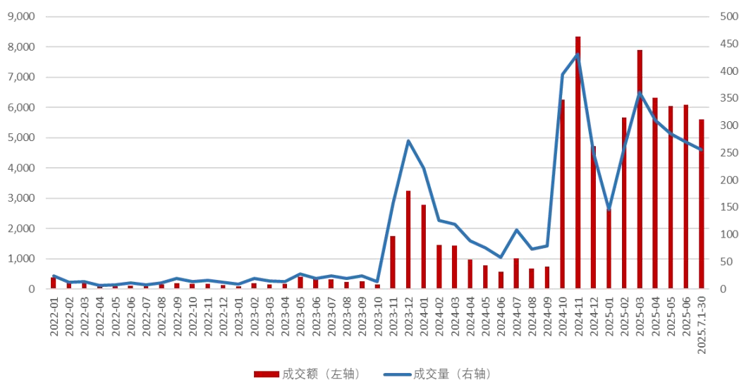
图 4：北交所成交量及成交额（单位：亿元，亿股）（截至 2025 年 7 月 30 日）
