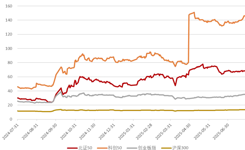
图 3: 市场主要板块 PE (截至 2025 年 7 月 30 日)
