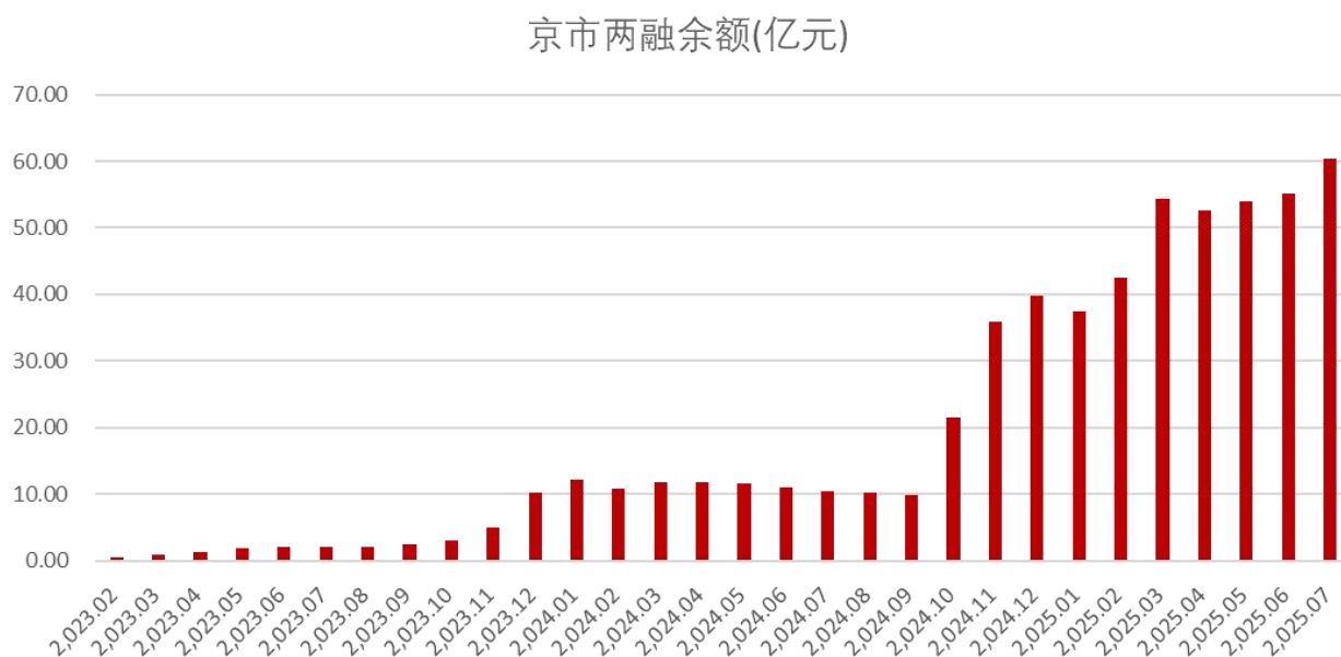
图 5：北交所融资融券余额及新增额（截至 2025 年 7 月 30 日）
