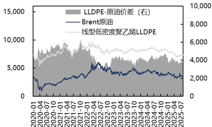
原油、聚乙烯LLDPE价格及价差（元/吨，元/吨）
