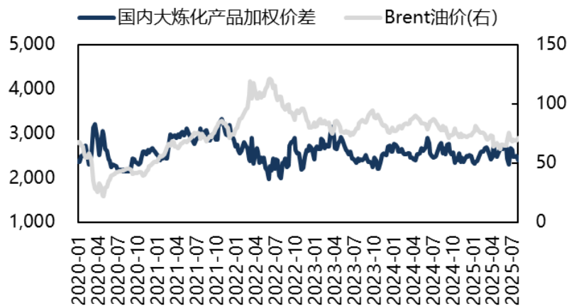
国内大炼化项目周度价差 (元/吨, 美元/桶)
