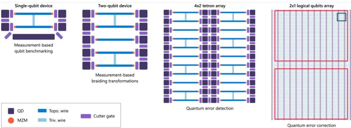
图表 利用tetrons实现容错量子计算的路线图
