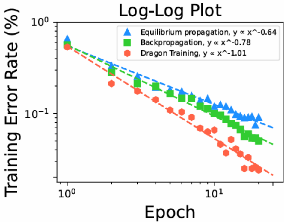
图表 训练方法性能对比（对数-对数坐标）
