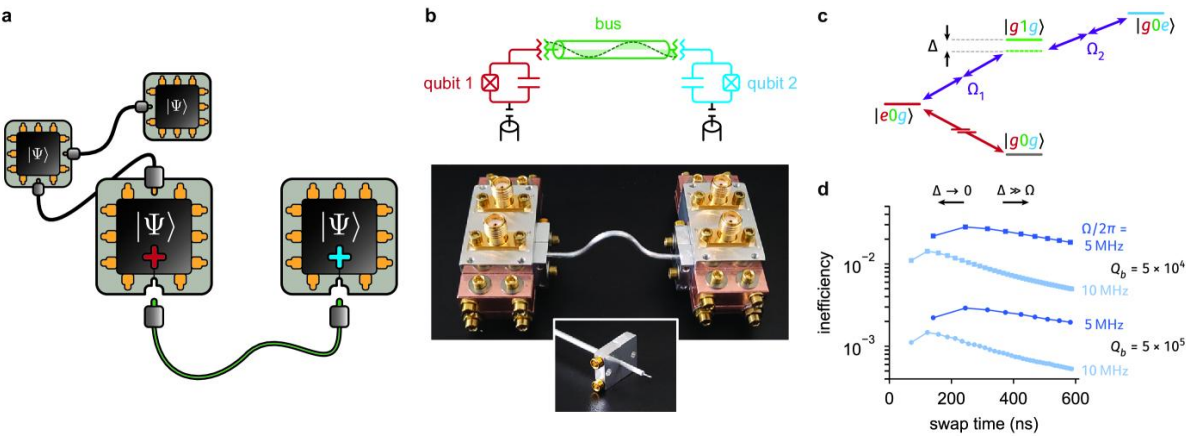
图表 实验概述，说明了将量子设备扩展为模块网络如何允许子系统的重新配置或更换，强调了通过可拆卸链路在不同模块中的量子比特之间高保真传输量子态的能力。
