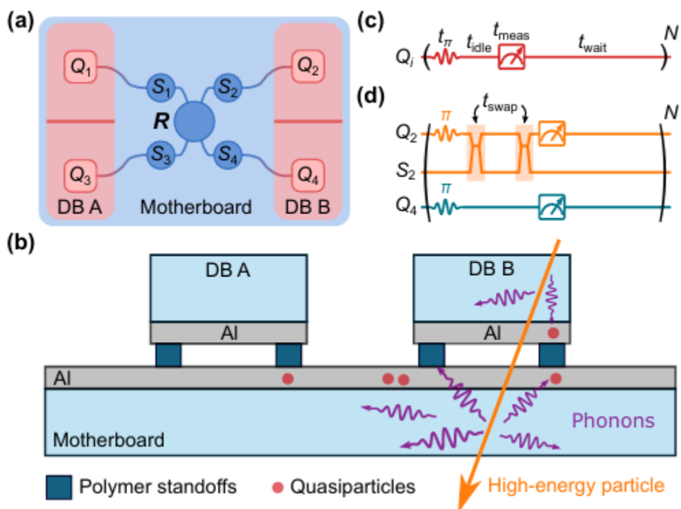
图表 模块化量子处理器的布局和测量脉冲序列
