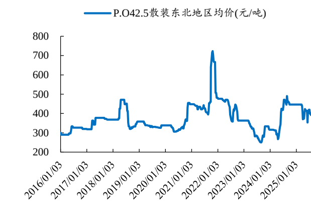
图10：本周东北地区水泥价格环比上涨 0.51%
