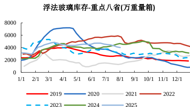
图37：重点八省浮法玻璃库存接近 2024 年同期水平
