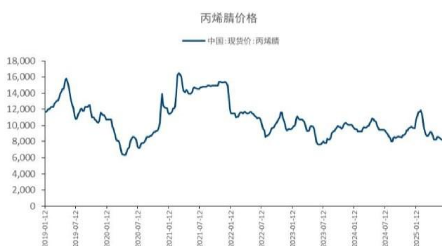
图3: 丙烯腈价格持平
