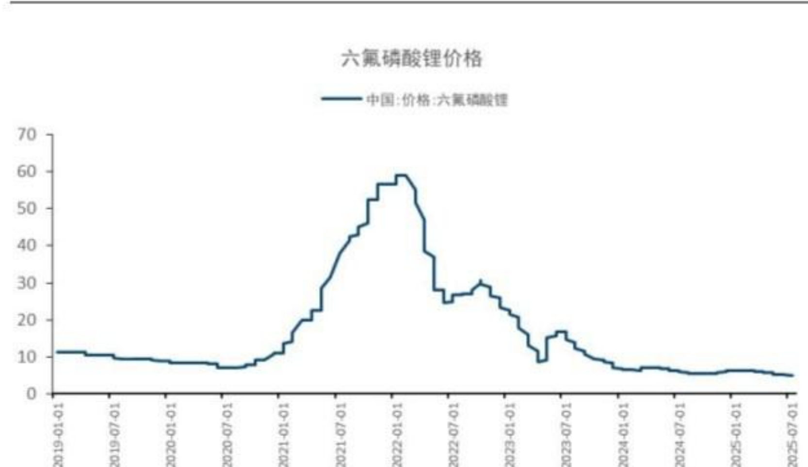
图6: 六氟磷酸锂价格上升
