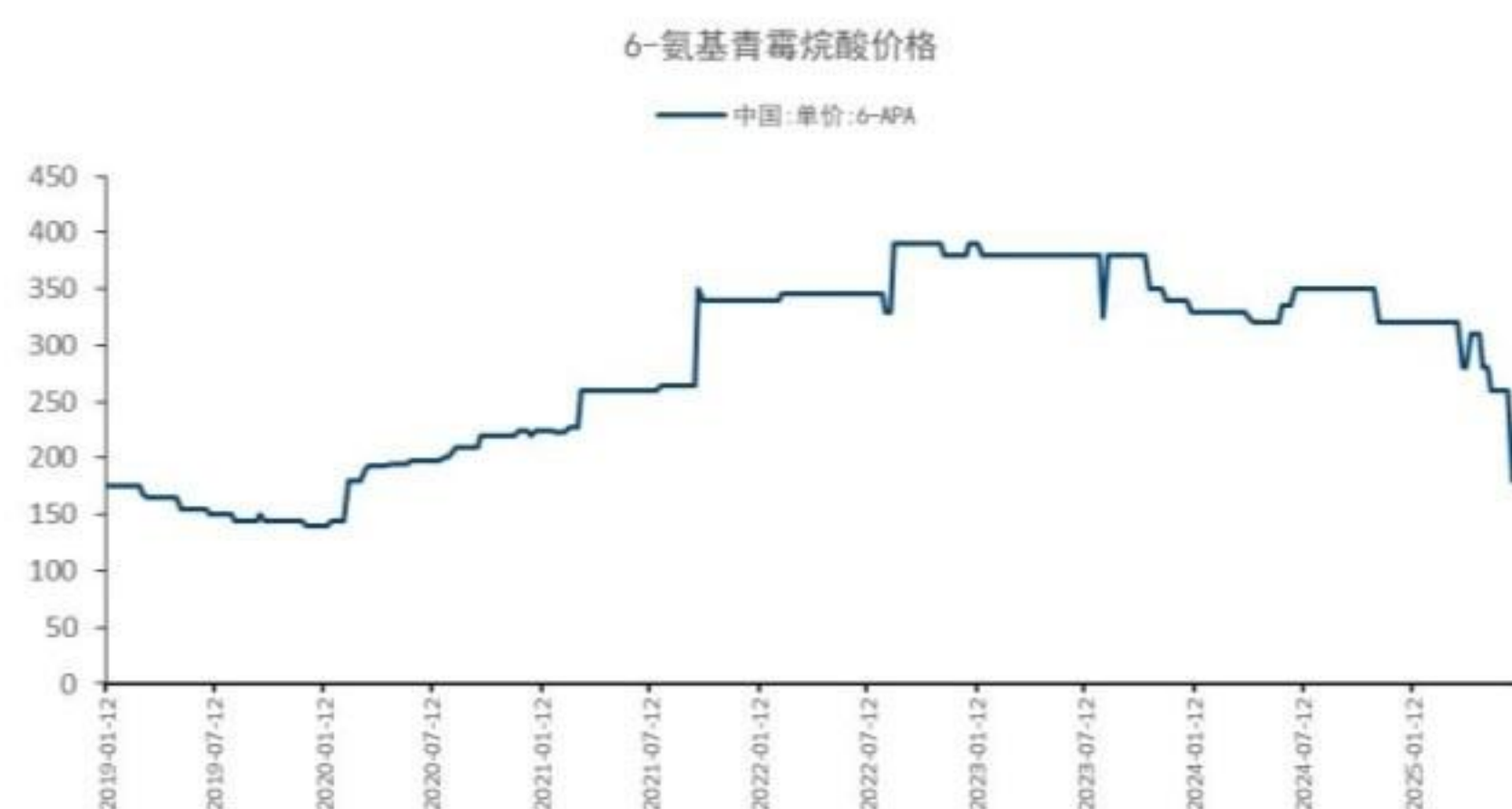
图2: 6-氨基青霉烷酸价格持平
