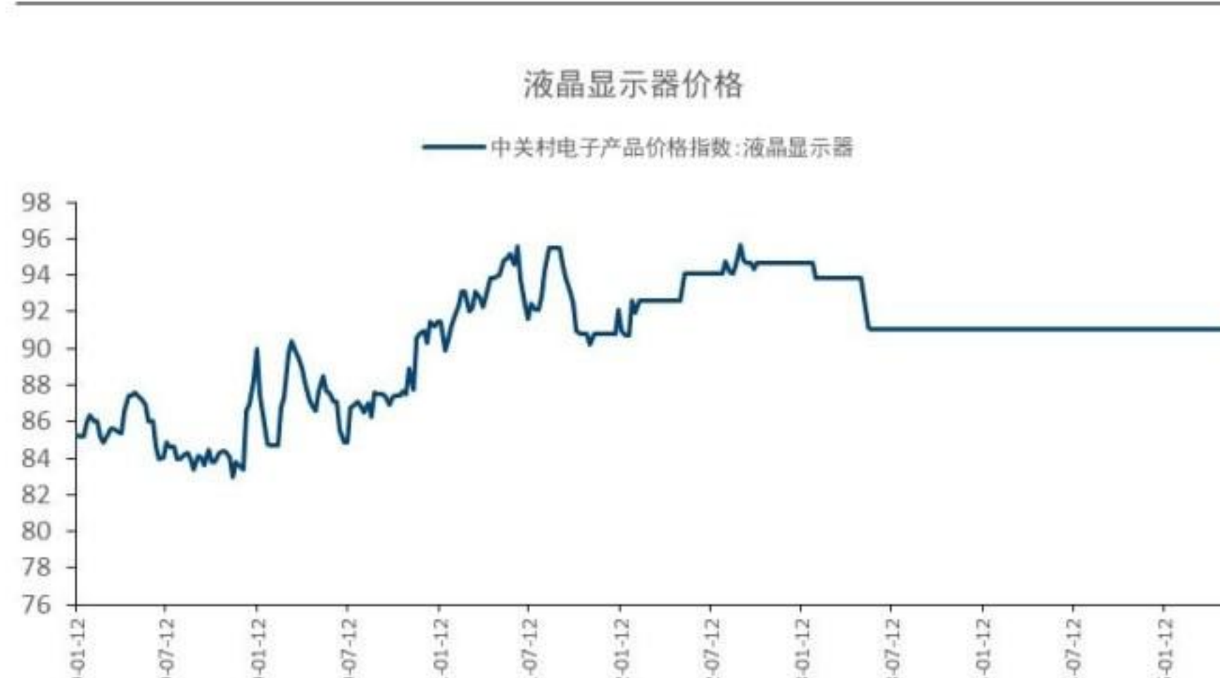
图7: 液晶显示器价格不变
