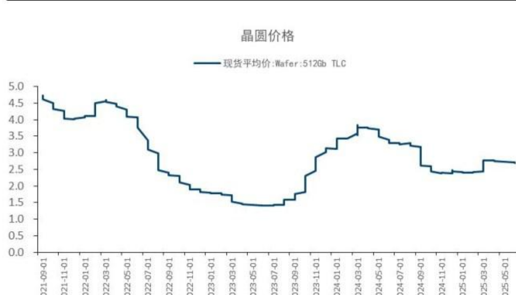
图5: 晶圆价格上升
