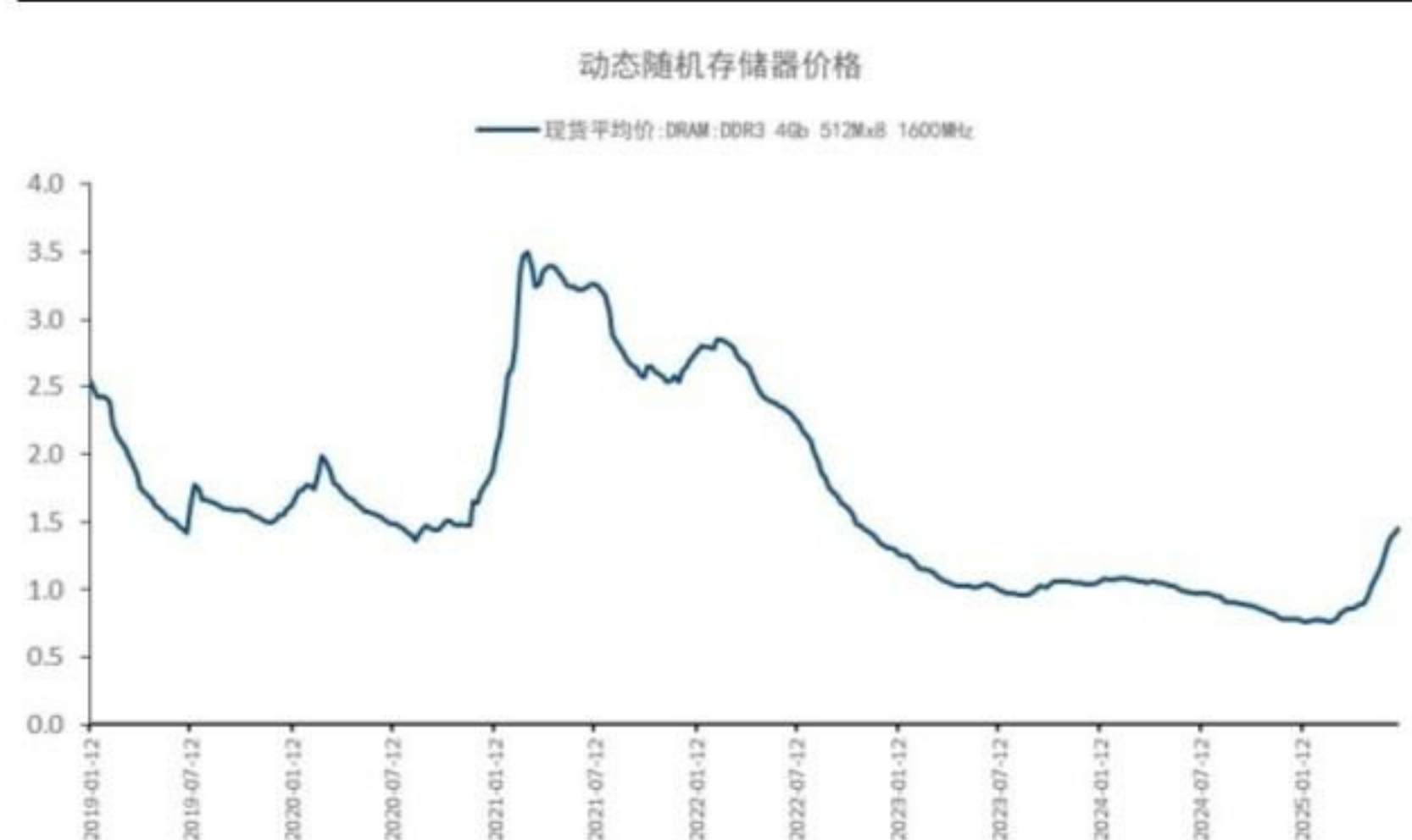
图4: 动态随机存储器价格上升
