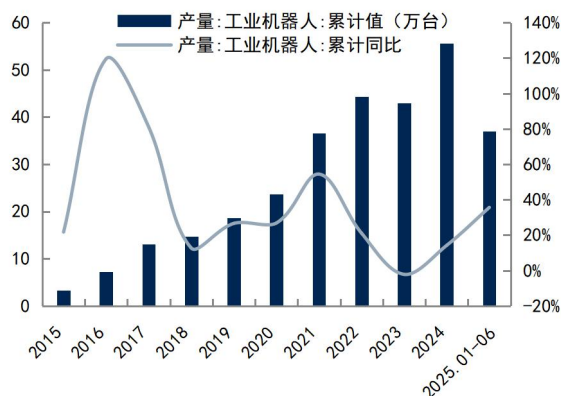
图23：2025 年 1-6 月中国工业机器人产量累计同比增长 35.60%
