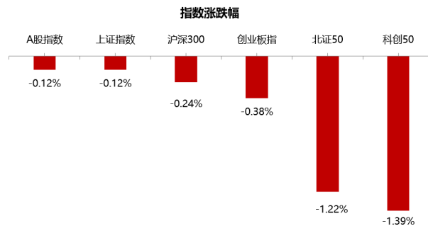
图2: 指数涨跌幅 (截至 2025/08/08)
