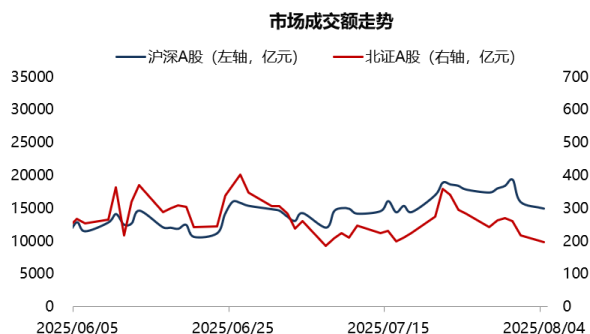
图1: 市场成交额走势 (截至 2025/08/08)
