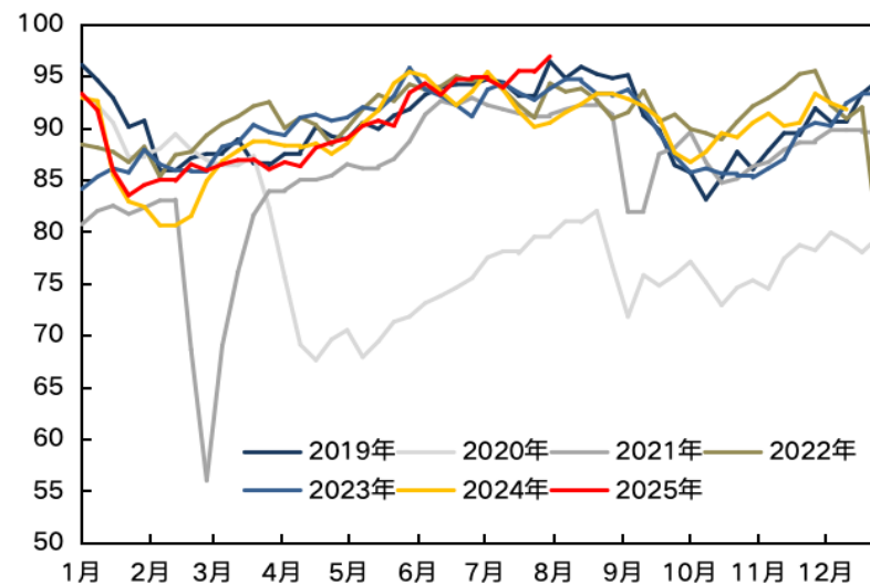
美国炼厂开工率 (%)
