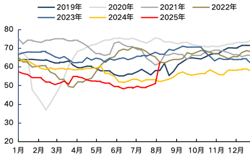
山东炼厂季节性开工率 (%)
