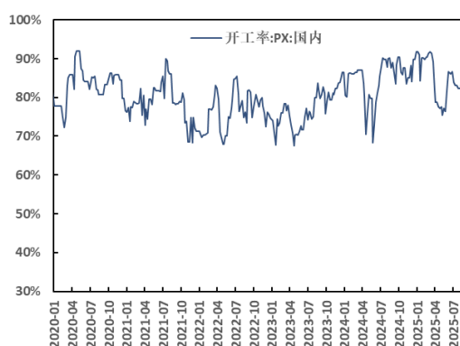
图 59: PX 开工率 (%)
