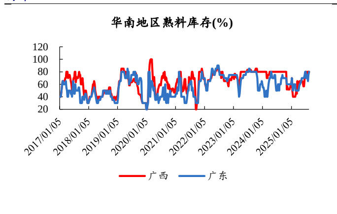
图17：本周华南地区熟料库存广东环比上升，广西环比持平
