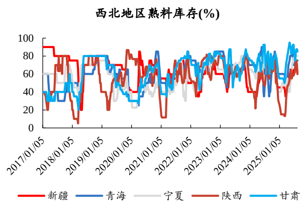
图23：本周西北地区新熟料库存陕西、甘肃环比下降，青海、新疆、宁夏环比持平
