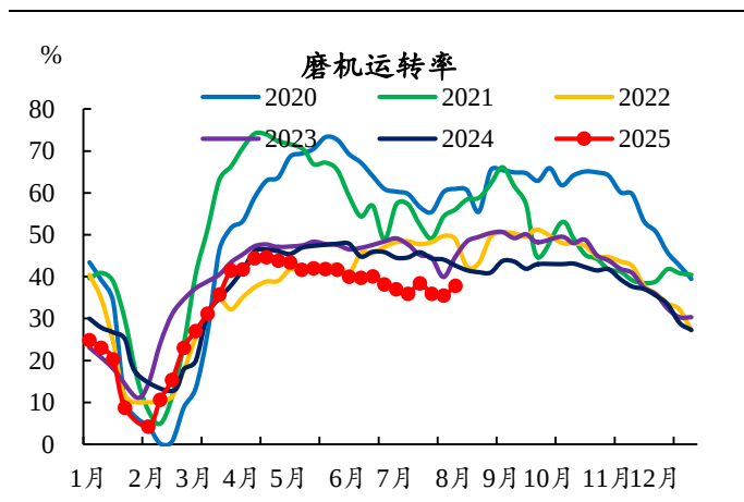
图3：磨机运转率环比回升
